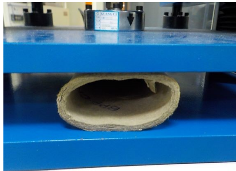
試験状態
