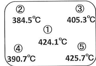
設定:High温度分布 Ave:406.06°C
