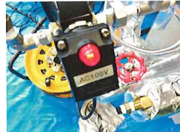
冷却水電磁弁AC100V
