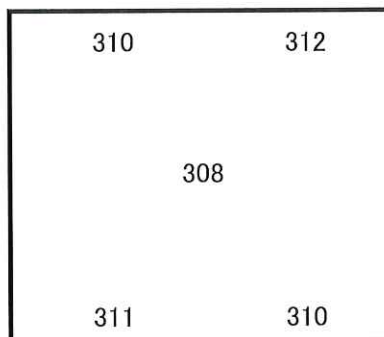
センター及び角から50mm弊社表面温度計測定(°C)
