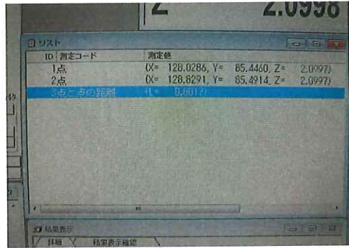
X方向測定及び結果:0.8017mm
