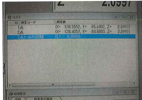
Y方向測定及び結果:0.8088mm
