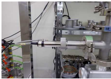
・測定子:ULVAC製 WP-01(社内用)
