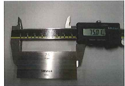
図4. 計測後表示75.01mm
